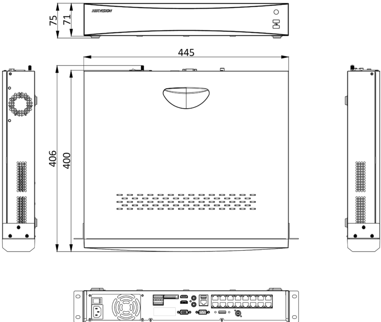
scale/1:1;Unit/mm
