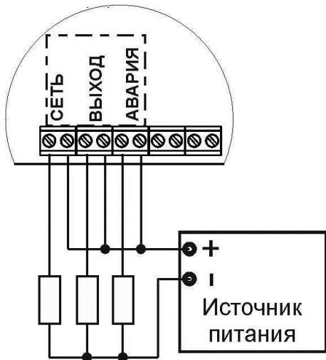
Рисунок 5 – Подключение внешних устройств автоматики
